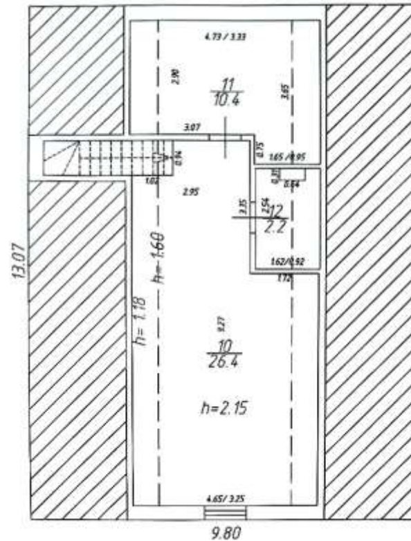
План 2 этажа
