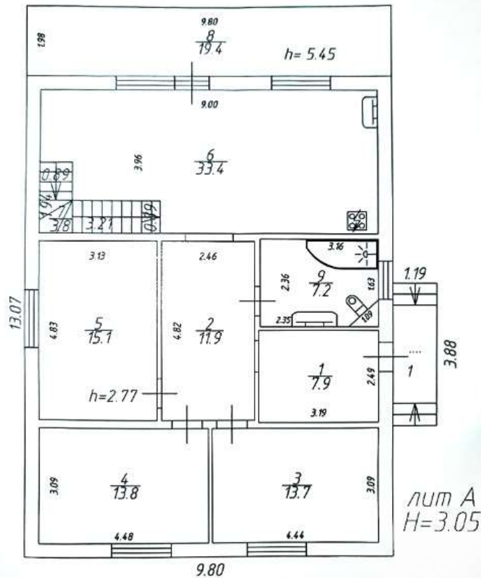
План 1 этажа
